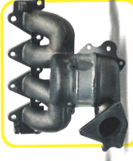
E. MANIFOLDS - integ. cat. izp. kolektorji - katalizator
